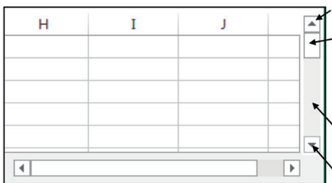
Die Bildlaufleisten
